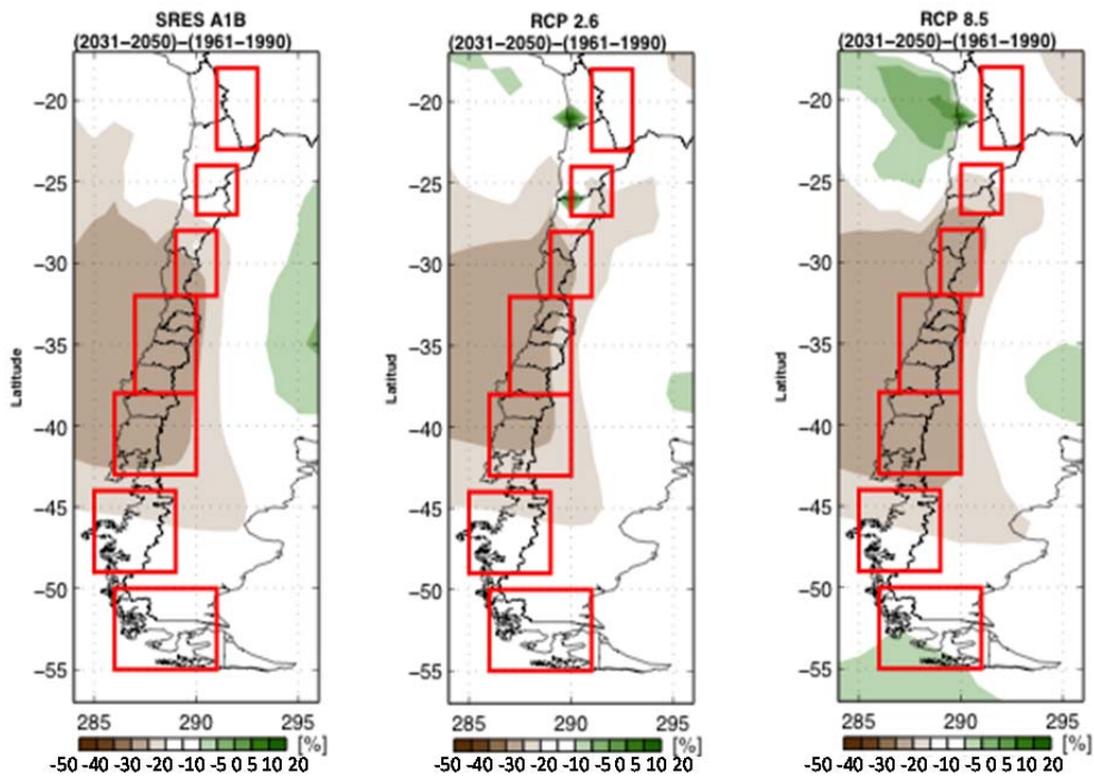
Figura 3. Proyecciones de precipitaciones periodo 2031-2050 (U. de Chile, 2012)
